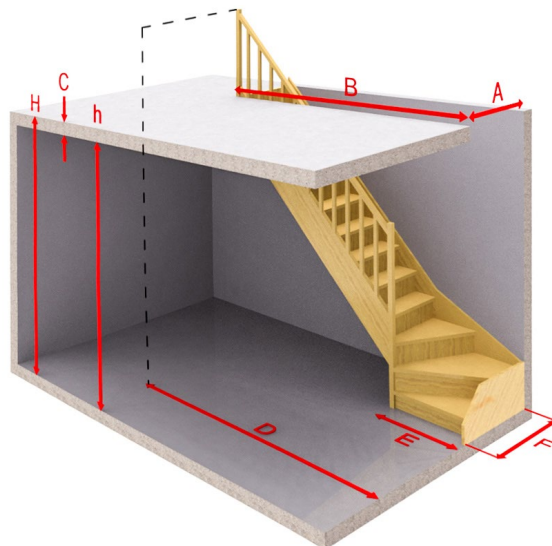
Ľavotočivé s dolným nábehom
